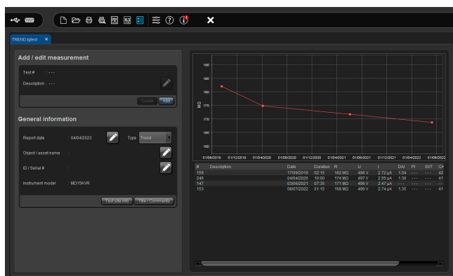
Análise de tendência (megôhmetros e micro-ohmímetros)
