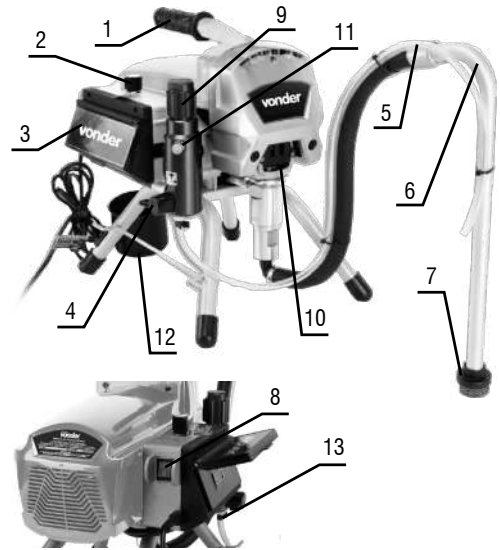
Fig. 1 – Componentes
