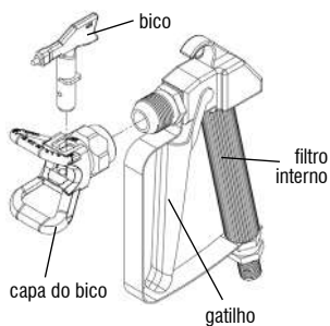
Fig. 2 – Componentes da pistola
